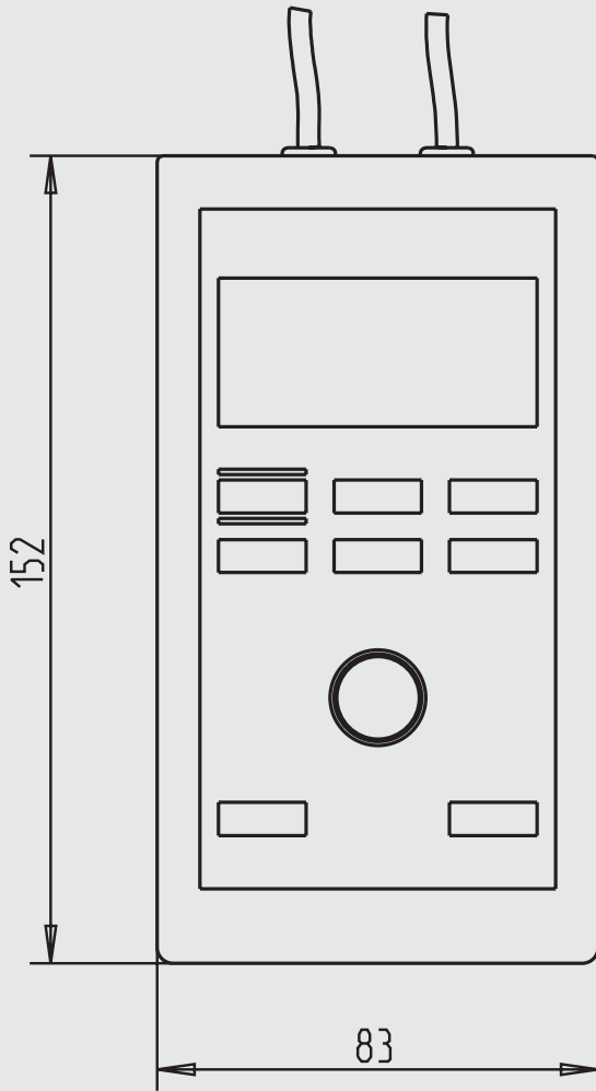
Frontansicht
